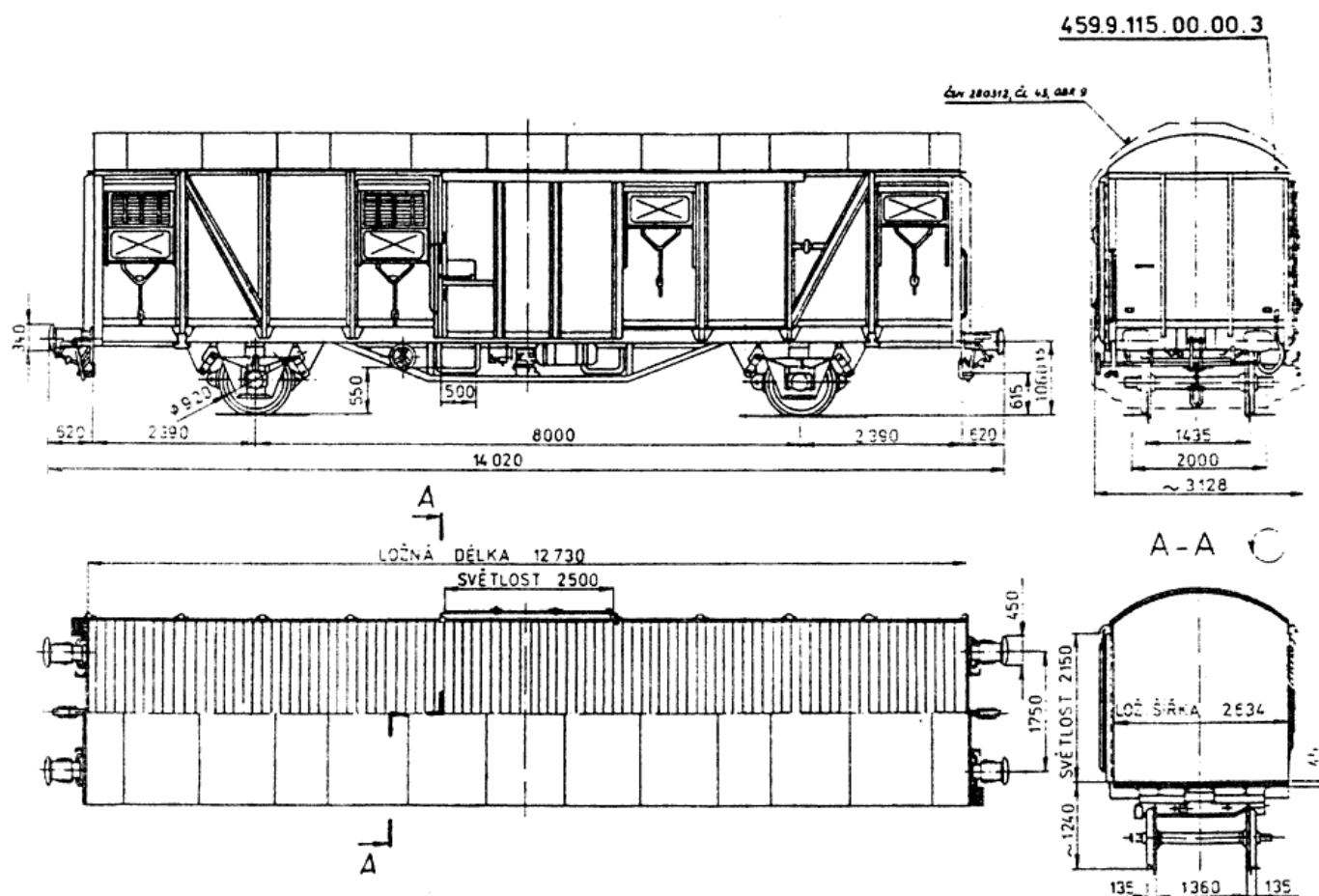
Obr. 2: Náčrt nákladního železničního vozu řady Gbkkqs/Ztscc12
