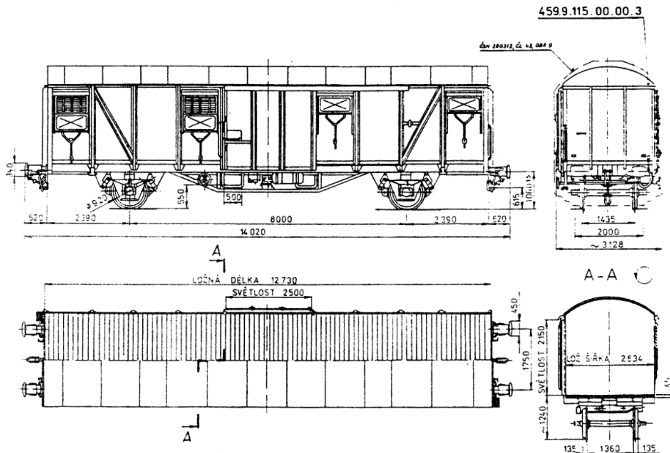
Obr. 2: Náčrty nákladního železničního vozu řady Gbkkqs/Ztscc12
